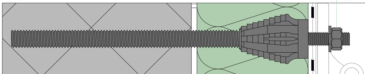
PARTICOLARE A
