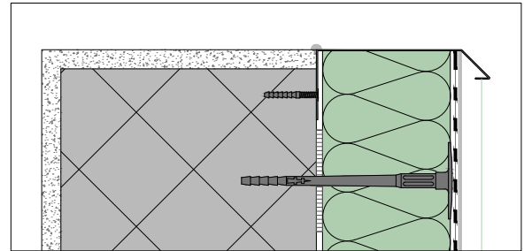
PARTICOLARE A
