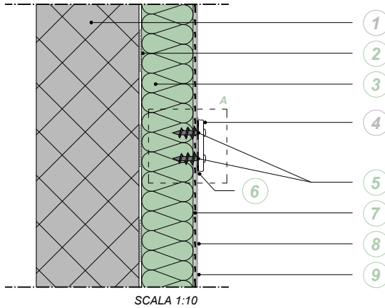
PARTICOLARE A
