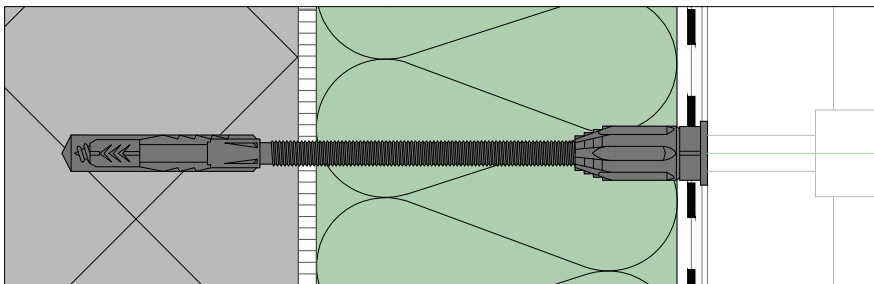
PARTICOLARE A
