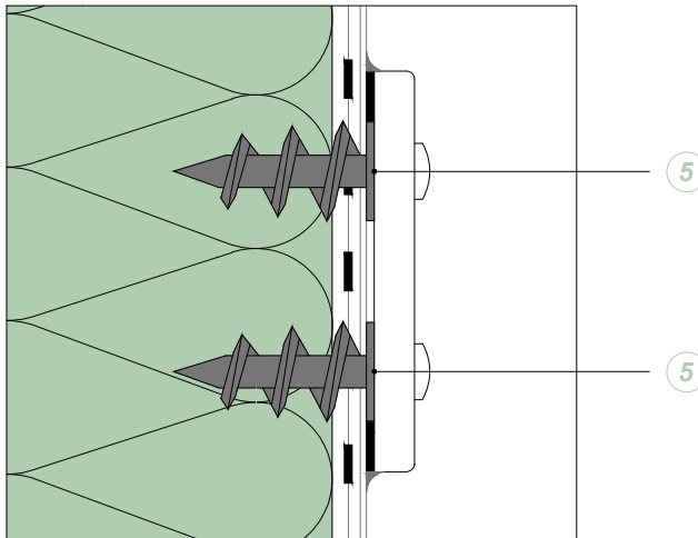
PARTICOLARE A
