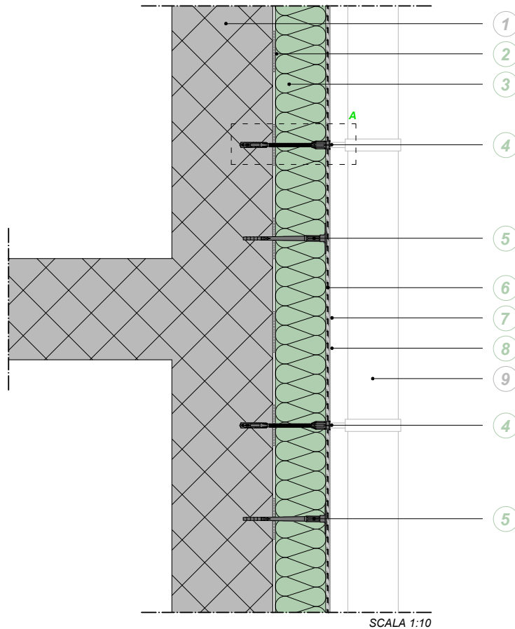
PARTICOLARE A
