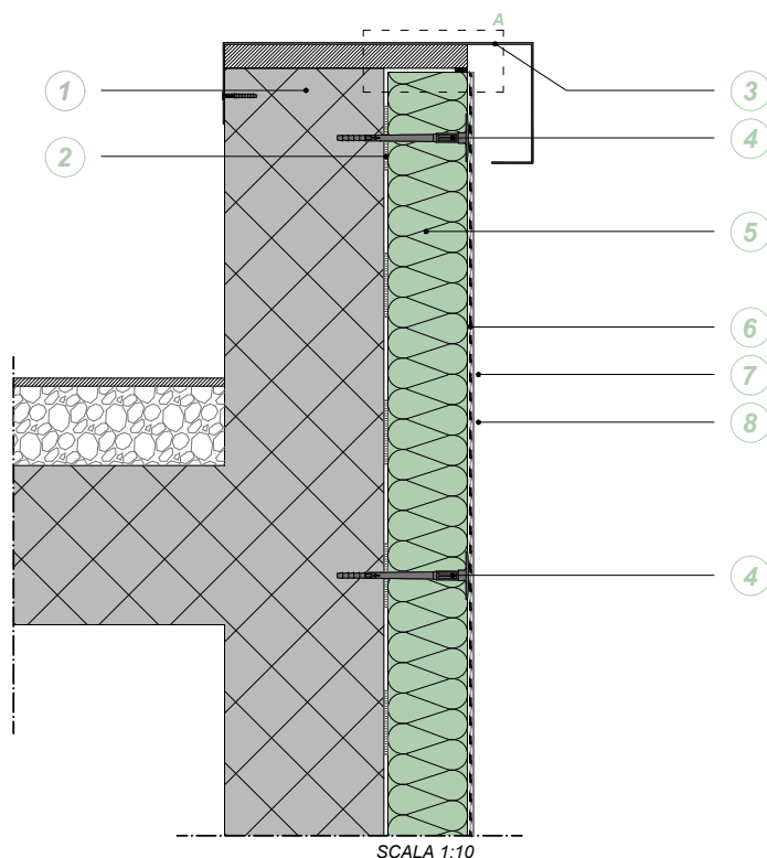
PARTICOLARE A
