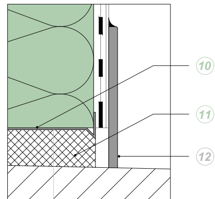
PARTICOLARE A SCALA 1:2
