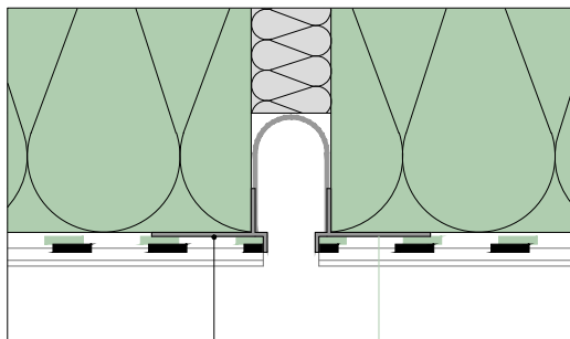
PARTICOLARE A
