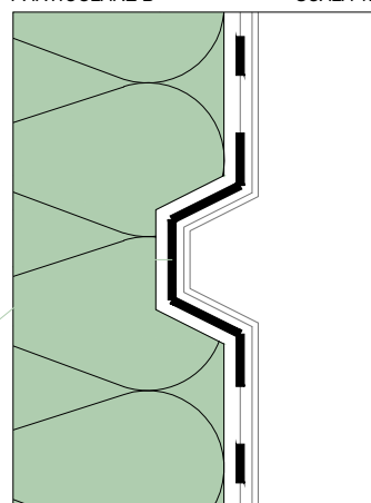
PARTICOLARE B SCALA 1:2
