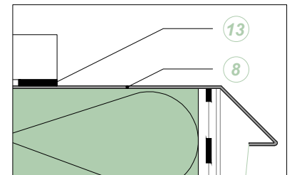
PARTICOLARE B
