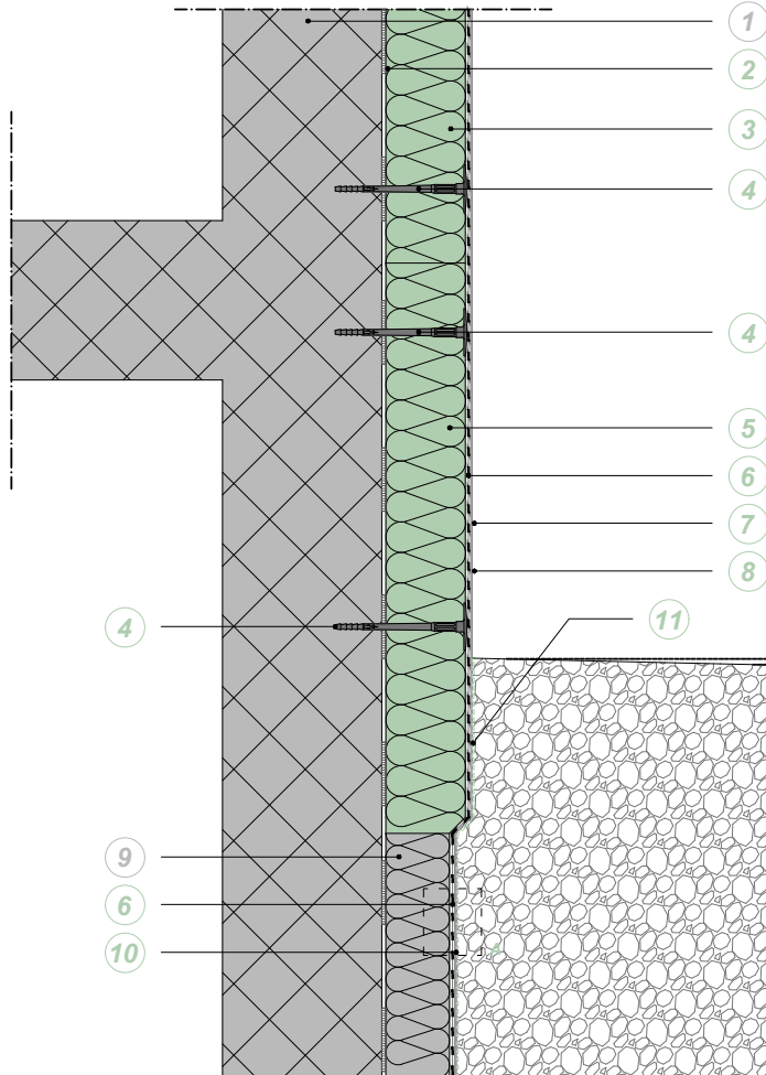
SCALA 1:10
