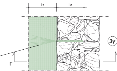
ΚΑΤΟΨΗ ΣΥΝΕΧΗΣ ΑΓΚΥΡΩΣΗ ΙΝΟΠΛΕΓΜΑΤΩΝ GEOSTEEL GRID 200/400 Ή RINFORZO ARV 100
