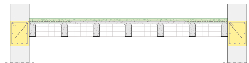
ΤΟΜΗ Α - Α' ΕΝΙΣΧΥΣΗ ΔΙΑΦΡΑΓΜΑΤΙΚΗΣ ΛΕΙΤΟΥΡΓΙΑΣ ΠΛΑΚΑΣ Ο.Σ (ΔΟΚΙΔΩΤΗΣ Ή ΟΛΟΣΩΜΗΣ) ΜΕ ΕΦΑΡΜΟΓΗ ΣΥΣΤΗΜΑΤΩΝ GEOLITE® FRC .
