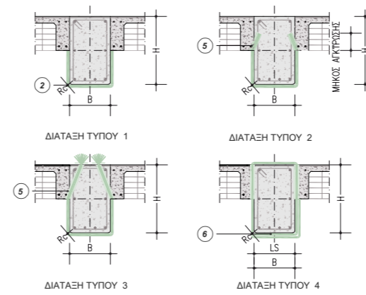
ΤΟΜΗ Α - Α' ΔΙΑΤΜΗΤΙΚΗ ΕΝΙΣΧΥΣΗ - ΔΙΑΤΑΞΕΙΣ ΧΑΛΥΒΔΟΥΨΑΣΜΑΤΩΝ
