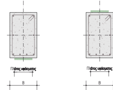
ΤΟΜΗ Α - Α' ΤΟΜΗ Β - Β' ΚΑΜΠΤΙΚΗ ΕΝΙΣΧΥΣΗ ΔΟΚΩΝ - ΕΦΑΡΜΟΓΗ ΧΑΛΥΒΔΟΥΦΑΣΜΑΤΩΝ ΣΤΗΝ ΑΝΩ ΚΑΙ ΚΑΤΩ ΠΑΡΕΙΑ
