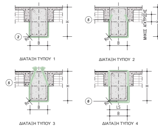
ΤΟΜΗ Α - Α' ΔΙΑΤΜΗΤΙΚΗ ΕΝΙΣΧΥΣΗ - ΔΙΑΤΑΞΕΙΣ ΧΑΛΥΒΔΟΥΨΑΣΜΑΤΩΝ
