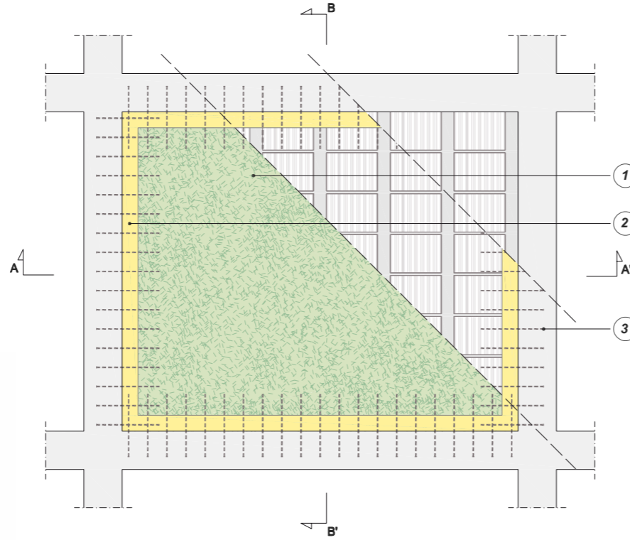
ΚΑΤΟΨΗ ΕΝΙΣΧΥΣΗ ΔΙΑΦΡΑΓΜΑΤΙΚΗΣ ΛΕΙΤΟΥΡΓΙΑΣ ΠΛΑΚΑΣ Ο.Σ (ΔΟΚΙΔΩΤΗΣ Ή ΟΛΟΣΩΜΗΣ) ΜΕ ΕΦΑΡΜΟΓΗ ΣΥΣΤΗΜΑΤΩΝ GEOLITE® FRC .
