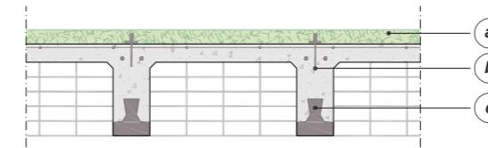
ΔΟΚΙΔΩΤΗ ΠΛΑΚΑ Ο.Σ
