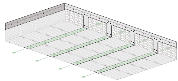
ΑΞΟΝΟΜΕΤΡΙΚΗ ΠΡΟΒΟΛΗ ΕΠΙΣΚΕΥΗ ΚΑΙ ΚΑΜΠΤΙΚΗ ΕΝΙΣΧΥΣΗ ΔΟΚΙΔΩΤΩΝ ΠΛΑΚΩΝ (ΑΠΕΙΚΟΝΙΖΕΤΑΙ Η ΚΑΤΩ ΠΑΡΕΙΑ)
