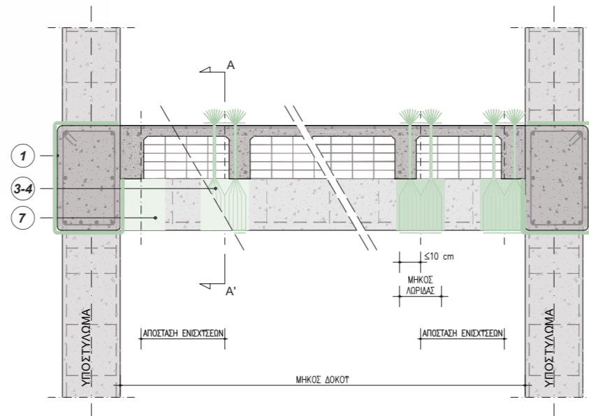
ΟΨΗ ΔΟΚΟΥ ΔΙΑΤΜΗΤΙΚΗ ΕΝΙΣΧΥΣΗ ΔΟΚΟΥ ΜΕ ΕΦΑΡΜΟΓΗ ΓΑΛΒΑΝΙΣΜΕΝΩΝ ΧΑΛΥΒΔΟΥΨΑΣΜΑΤΩΝ ΣΕ ΑΠΟΣΤΑΣΕΙΣ
