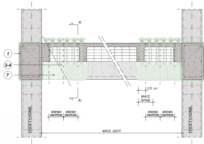
ΟΨΗ ΔΟΚΟΥ ΔΙΑΤΜΗΤΙΚΗ ΕΝΙΣΧΥΣΗ ΔΟΚΟΥ ΜΕ ΣΥΝΕΧΗ ΕΦΑΡΜΟΓΗ ΓΑΛΒΑΝΙΣΜΕΝΩΝ ΧΑΛΥΒΔΟΥΨΑΣΜΑΤΩΝ
