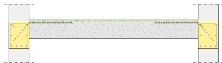
ΤΟΜΗ Β - Β' ΕΝΙΣΧΥΣΗ ΔΙΑΦΡΑΓΜΑΤΙΚΗΣ ΛΕΙΤΟΥΡΓΙΑΣ ΠΛΑΚΑΣ Ο.Σ (ΔΟΚΙΔΩΤΗΣ Ή ΟΛΟΣΩΜΗΣ) ΜΕ ΕΦΑΡΜΟΓΗ ΣΥΣΤΗΜΑΤΩΝ GEOLITE® FRC .
