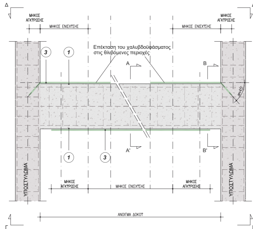
ΟΨΗ ΔΟΚΟΥ ΚΑΙ ΥΠΟΣΤΥΛΩΜΑΤΩΝ ΚΑΜΠΤΙΚΗ ΕΝΙΣΧΥΣΗ ΔΟΚΟΥ ΜΕ ΕΦΑΡΜΟΓΗ ΧΑΛΥΒΔΟΥΦΑΣΜΑΤΩΝ ΣΤΗΝ ΑΝΩ ΚΑΙ ΚΑΤΩ ΠΑΡΕΙΑ
