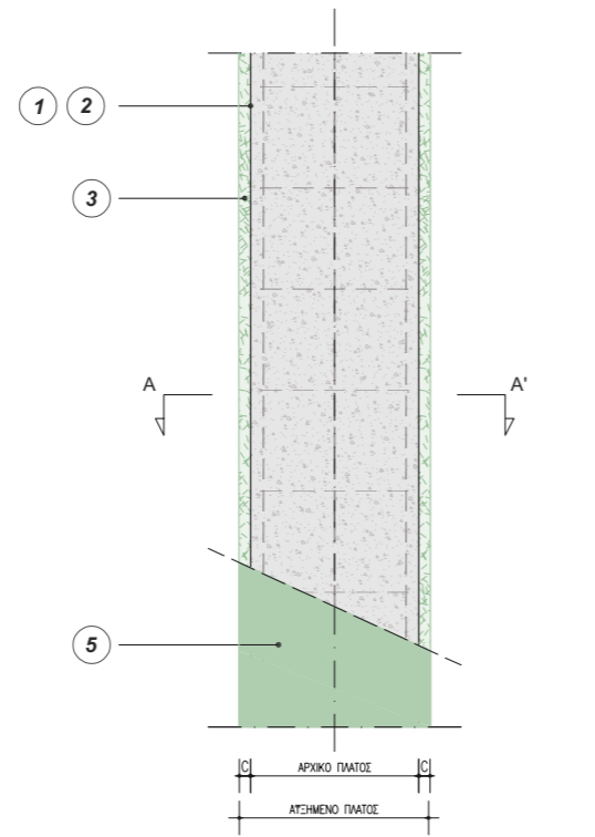
ΟΨΗ ΥΠΟΣΤΥΛΩΜΑΤΟΣ ΕΝΙΣΧΥΣΗ ΜΕ ΚΑΤΑΣΚΕΥΗ ΜΑΝΔΥΑ - ΣΥΣΤΗΜΑΤΟΣ ΙΝΟΠΛΙΣΜΕΝΟΥ ΣΚΥΡΟΔΕΜΑΤΟΣ GEOLITE® FRC
