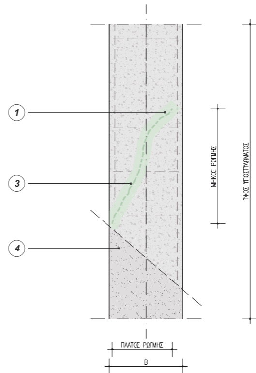
ΟΨΗ ΑΠΟΚΑΤΑΣΤΑΣΗΣ ΡΩΓΜΩΝ - ΑΡΜΟΛΟΓΗΣΗ ΜΕ ΡΗΤΙΝΗ
